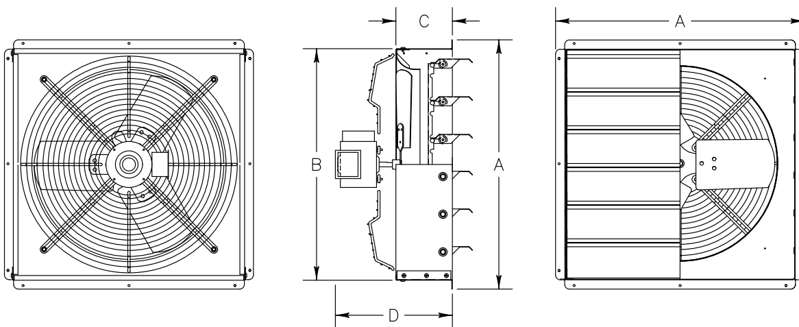
GPX Fan Dimensions
